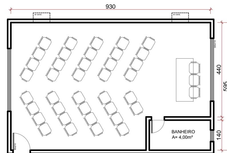
SALA MARITACA LAYOUT ESPINHA DE PEIXE ESCALA 1/50
