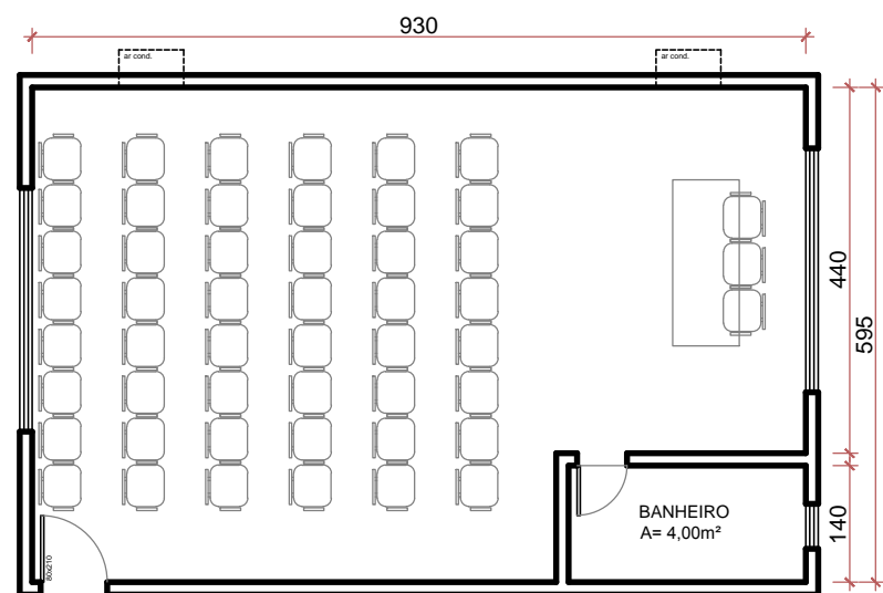
SALA MARITACA LAYOUT AUDITÓRIO ESCALA 1/50
